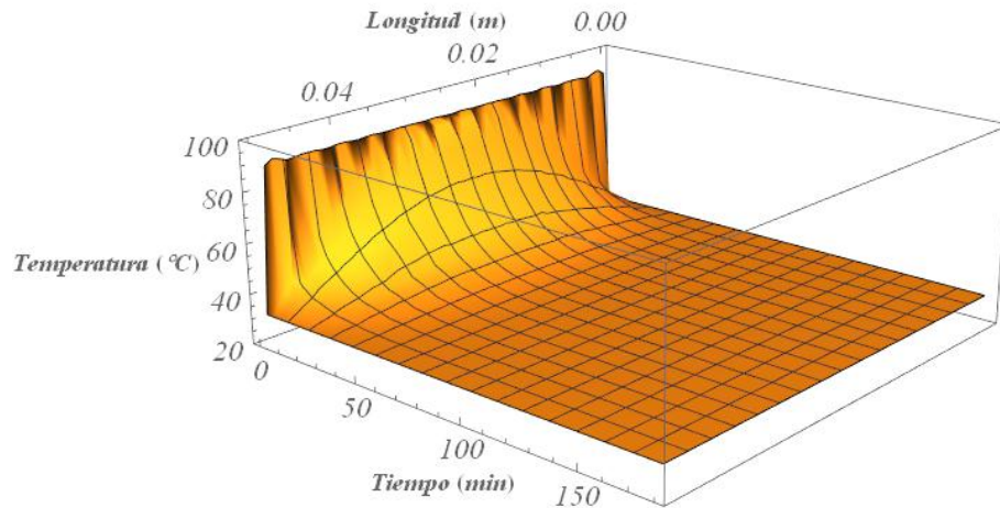
Figura 4. Gráfica de evolución de temperatura, para una de las caras de un cubo sólido ideal con las 6 caras sometidas a la misma temperatura constante T_0 .
